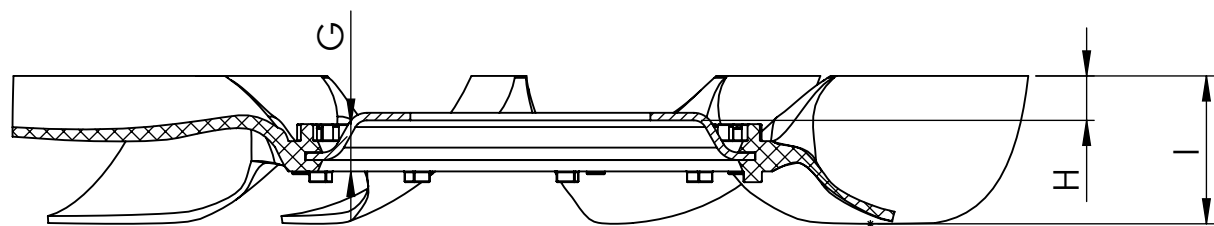
SECCIÓN A-A
