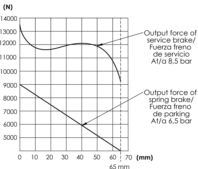
Force diagram / Diagrama de fuerzas
