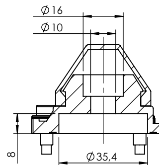
SECTION/SECCIÓN A-A
