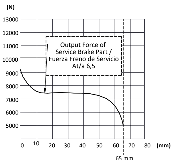
Force diagram / Diagrama de fuerzas
