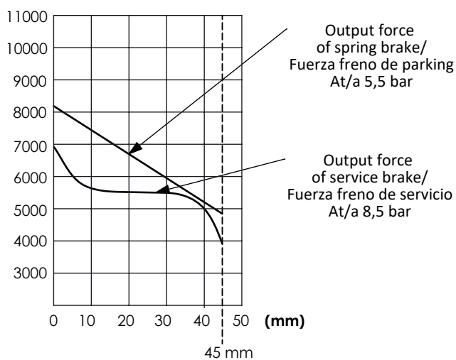
(N) Force diagram / Diagrama de fuerzas
