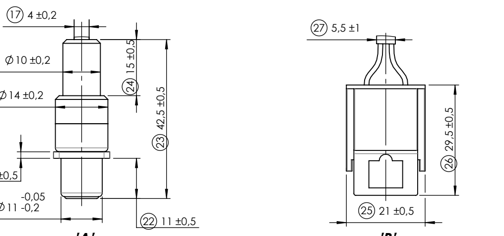
Scale / Escala 1 : 1 Hall sensor & inductive sensor / Sensor hall & sensor inductivo Scale / Escala 1 : 1 Position sensor connectors / Conectores de los sensores de posición
